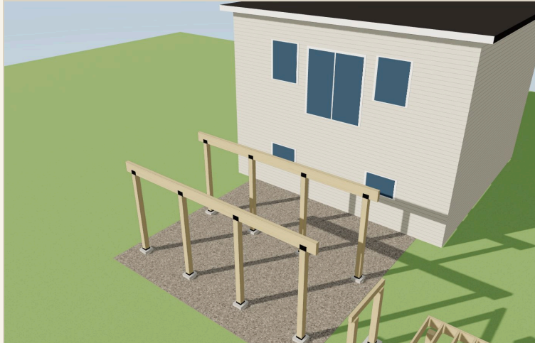
Step 4 · Beams — DROP 4x12 DF (4 posts) · DROP 4x12 DF (4 posts)
